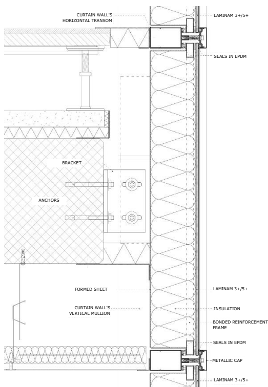
Вертикальный разрез
